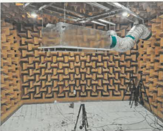
<소음 시험>
